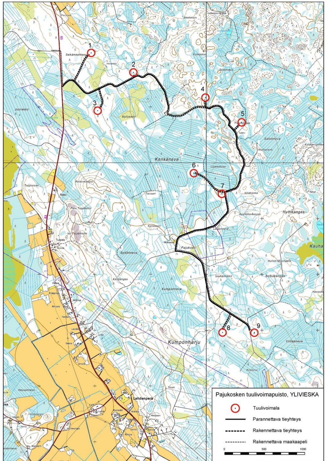
Kartta 4. Pajukosken tuulivoimapuiston voimaloiden, maakaapeleiden ja tieyhteyskijien sijainnit. Ei mittakaavassa.
