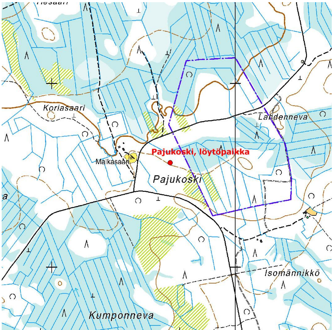
Kartta 5. Löytöpaikan Pajukoski sijainti (Muinaisjäännösrekisterin perusteella). MK 1 : 10 000.
