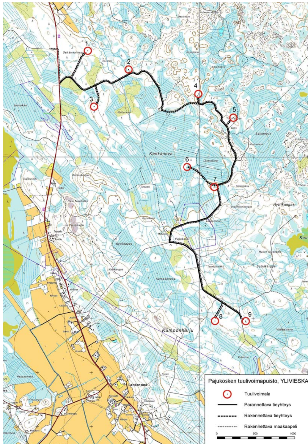
Kuva 2. Hankkeen alustava voimalasijoittelu, huoltotiestä ja sähkönsiirto.
