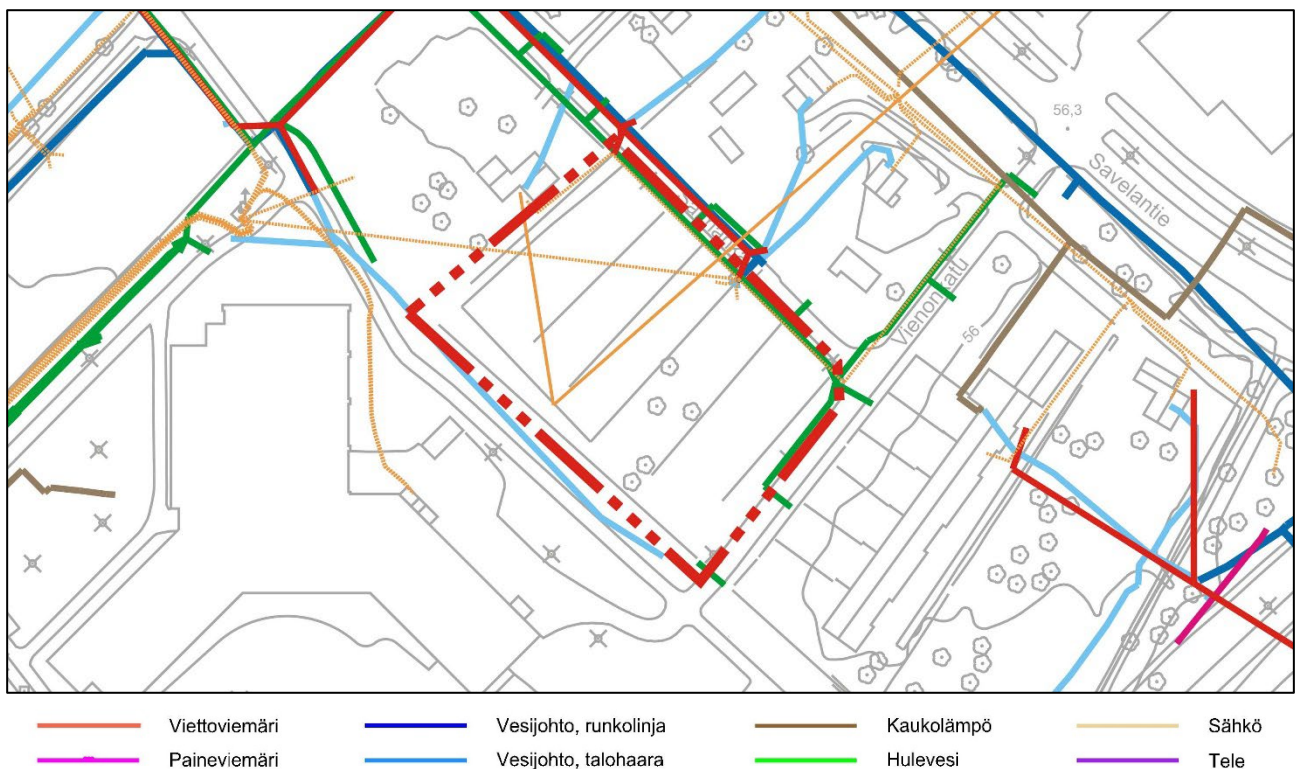
Kuva 12. Suunnittelualueen rakennettu kunnallistekniikka 29.8.2023.
