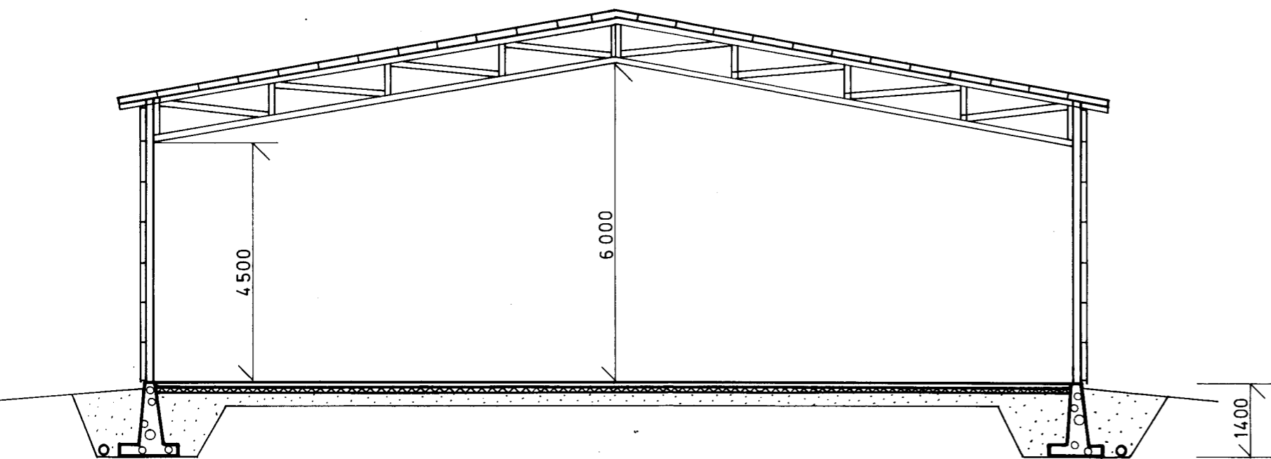
LEIKKAUS A-A 1:100
