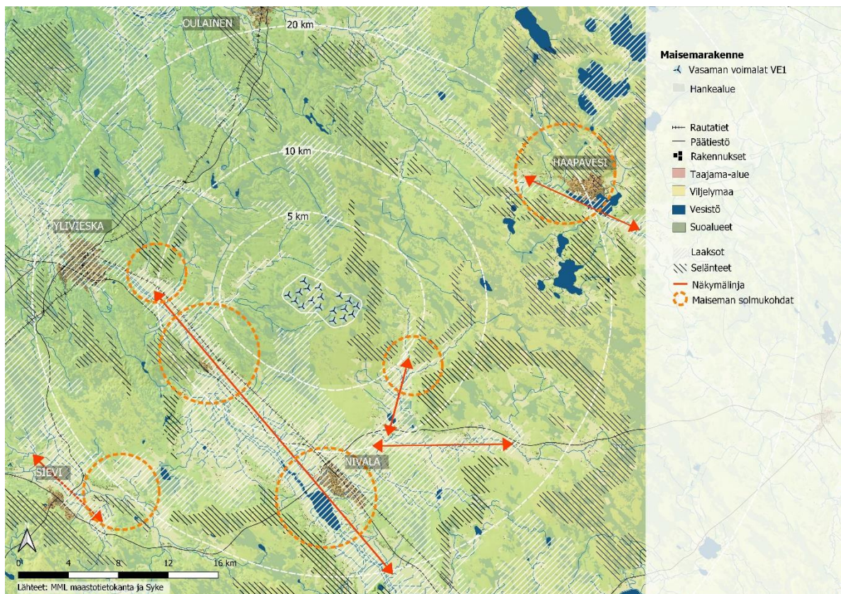
Kuva 2.4 Maisemarakenne: selänneet ja laaksot. Maiseman solmukohdat ja tärkeimmät näkymälinjat sijoittuvat Haapaveden taajamaan, Nivalan jokilaaksoon, Vähäkankaalle, Raudaskylän ja Isokosken välille, Järvikylään sekä Sarjakylän tienoille.
