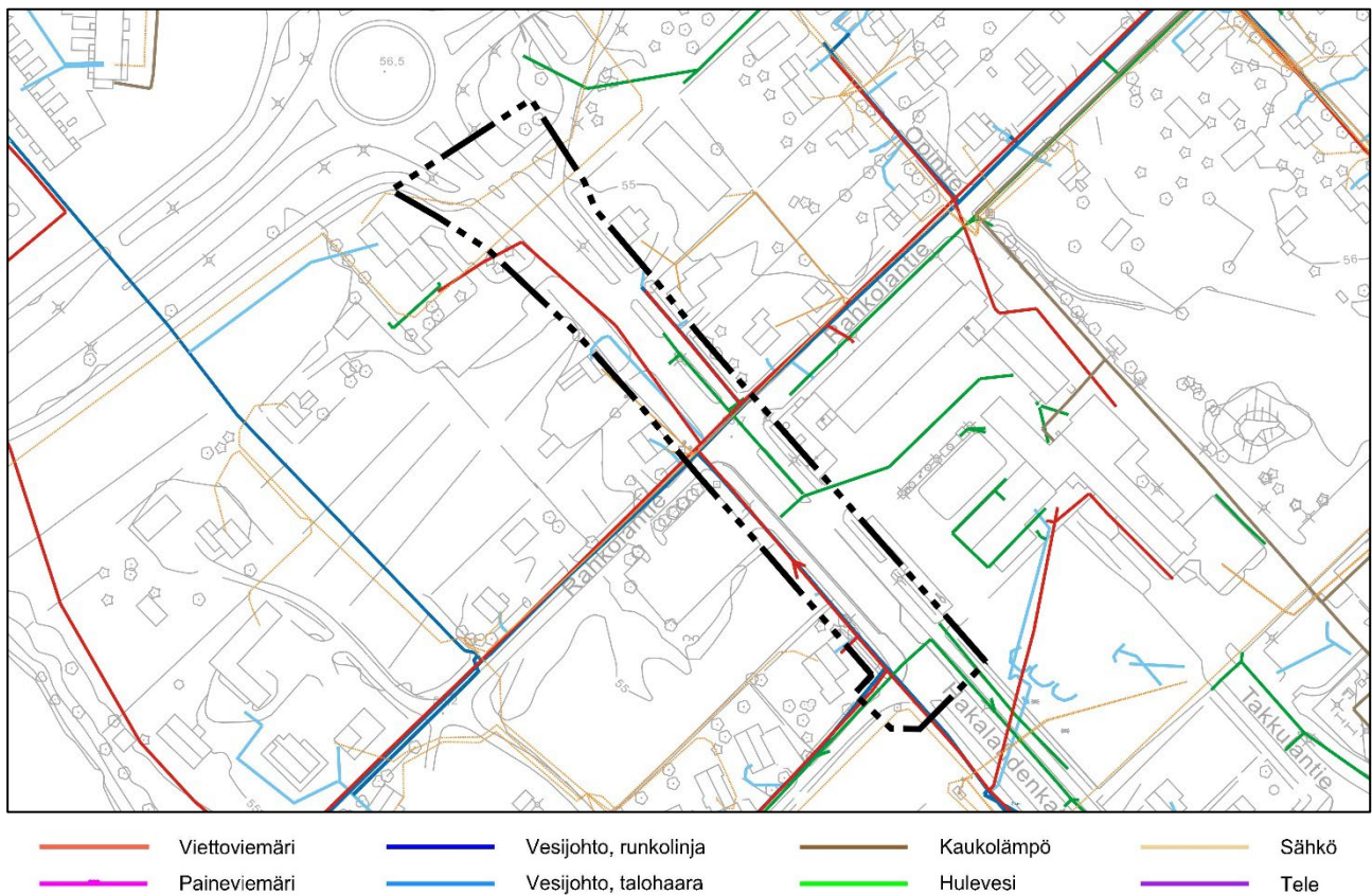
Kuva 11. Suunnittelualueen rakennettu kunnallistekniikka 15.9.2025.
