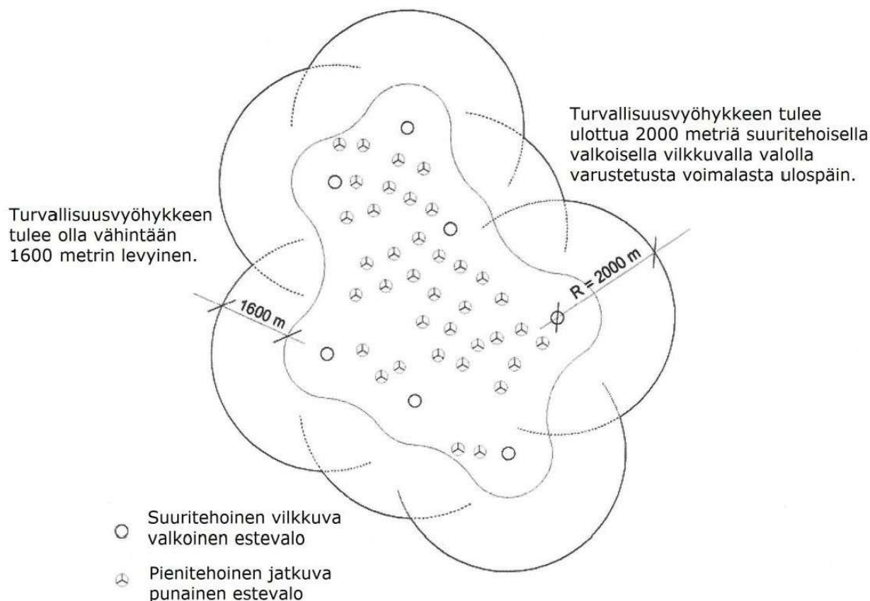
Kuva 70. Lentoestevalojen sijoitteluesimerkki, kun tuulivoimapuiston voimaloiden korkein pyyhkäisykohta on yli 150 metriä maanpinnasta. Tuulivoimaloiden ulkokehän muodostavat suuritehoiset B-tyypin vilkkuvat valkoiset lentoestevalot (Kuva Traficom).
