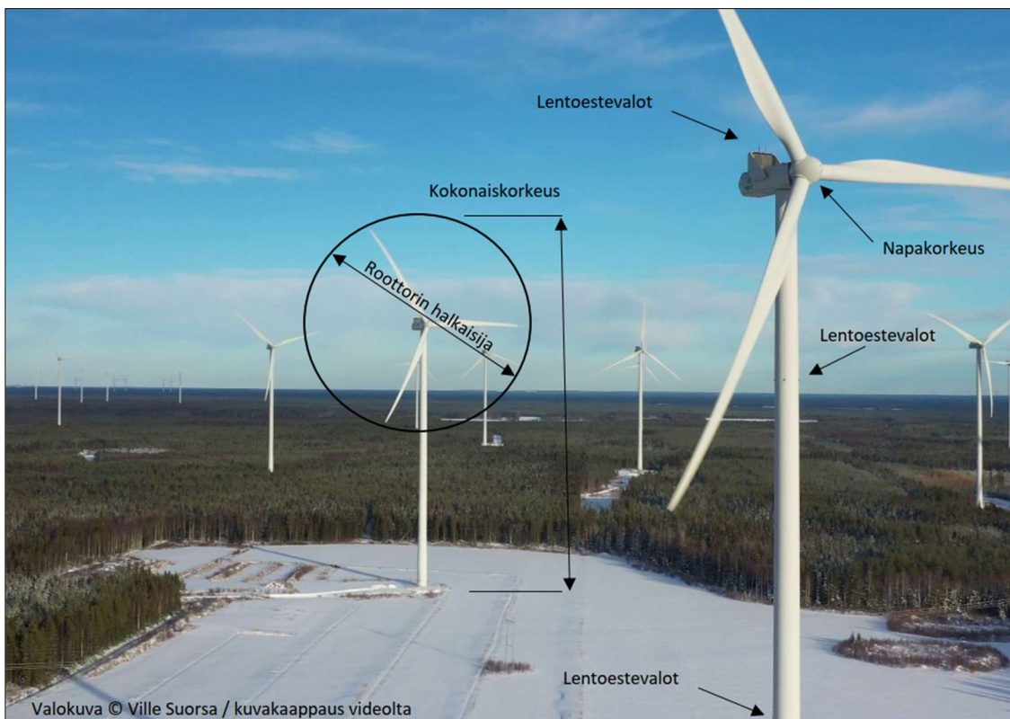
Kuva 68. Tuulivoimasanastoa. Valokuvan voimaloiden napakorkeus 140 metriä ja roottorin halkaisija 120 metriä, eli kokonaishkorkeus on 200 metriä. Verkasaloon tarkasteltavan voimalan maksimikokonaishkorkeus on noin 320 metriä.
