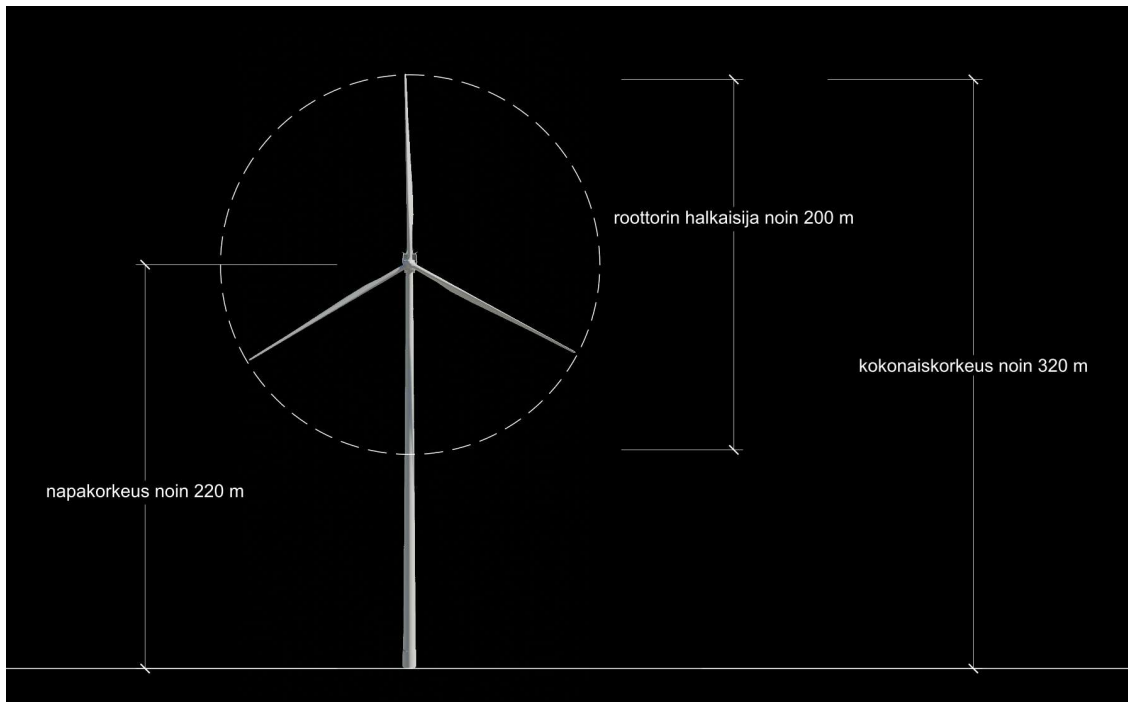
Kuva 67. Verkasaloon suunniteltujen voimaloiden napakorkeus on noin 220 metriä, roottoriympyrän halkaisija noin 200 metriä ja kokonaishkorkeus noin 320 metriä.
