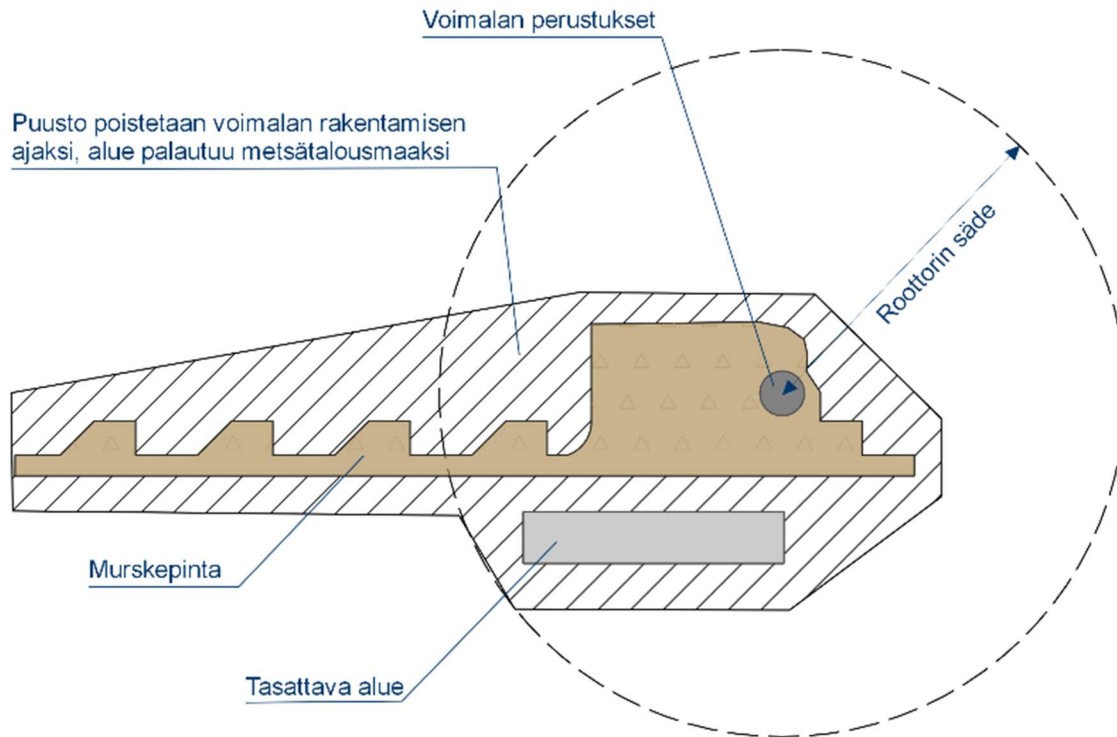
Kuva 74. Tyypillinen tuulivoimalan kokoamis- ja pystytysalue.
