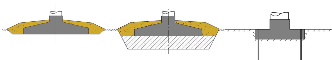
Kuva 71. Tuulivoimalat voidaan perustaa useilla eri tavoilla. Periaatekuvat maavaraisesta teräsbetoniperustuksesta, teräsbetoniperustuksesta massanvaihhdolla sekä kallioankkuroidusta teräsbetoniperustuksesta.
