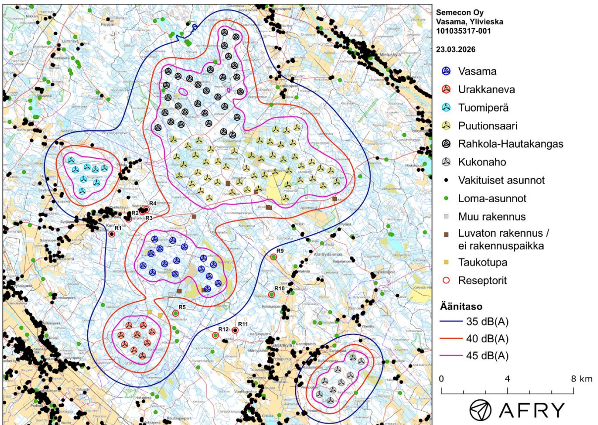
Kuva 3-2: Keskiäänitasot LAeq, kun mallinnoissa huomioidaan Vasaman sekä läheisten tuulivoimalapais- tojen voimat.
