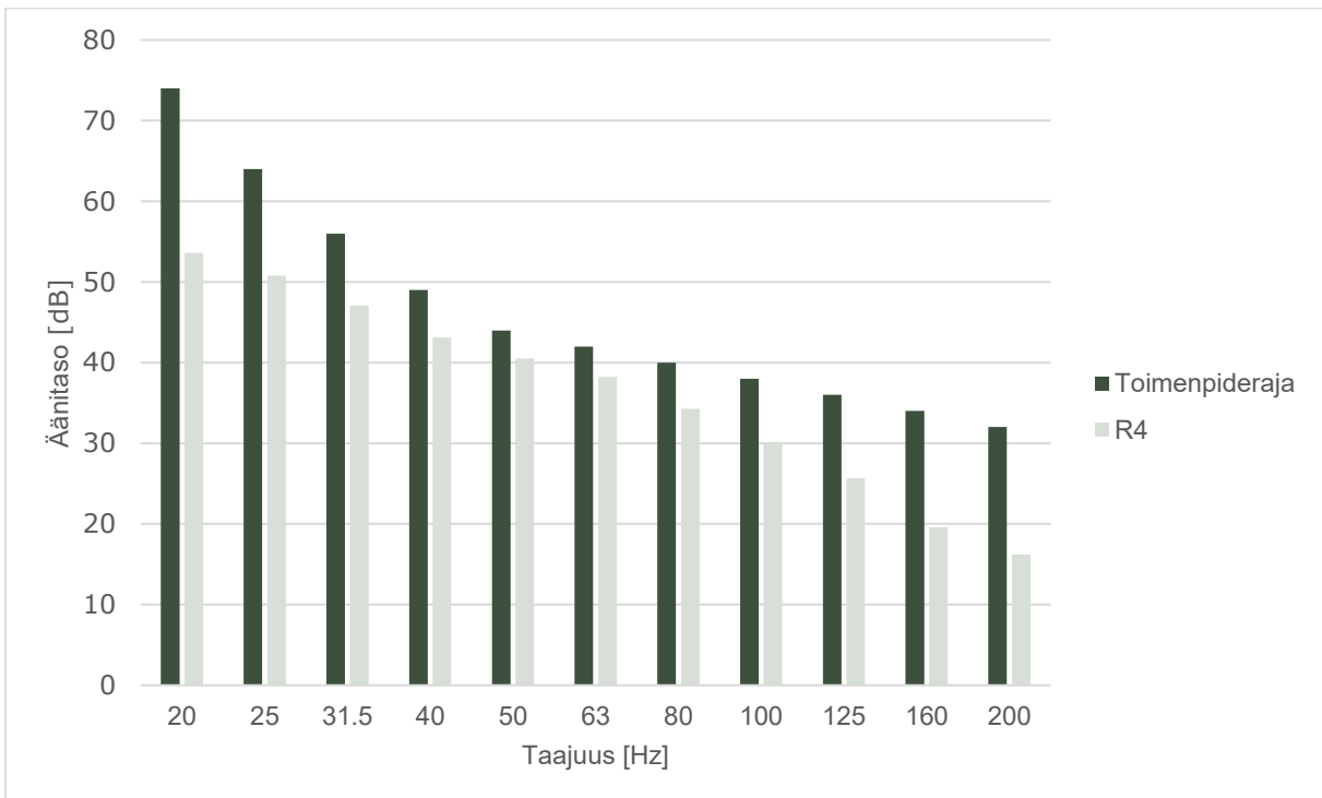
Kuva 3-3: Matalataajuisten sisämelun tasot reseptorin R4 kohdalla.
